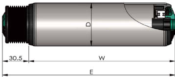
多楔带输送辊筒
