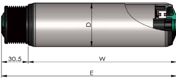
多楔带输送辊筒
