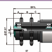
3224 Double polymer sprocket
