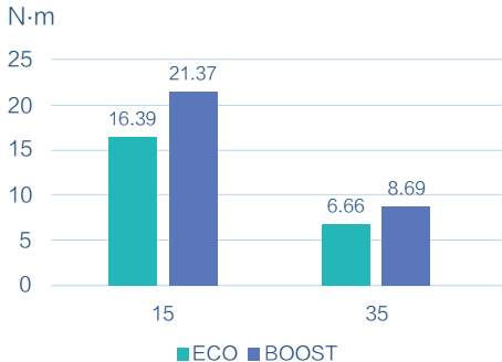
ECO和BOOST的启动扭矩对比
