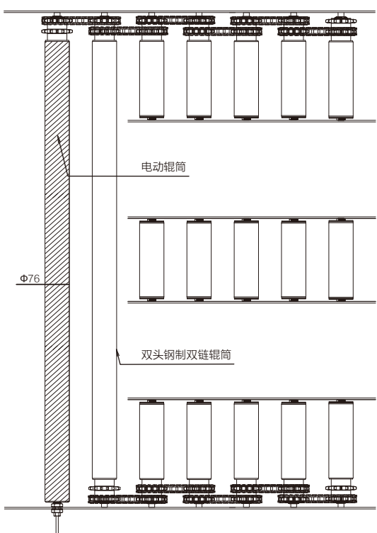
多排短辊筒应用示意
