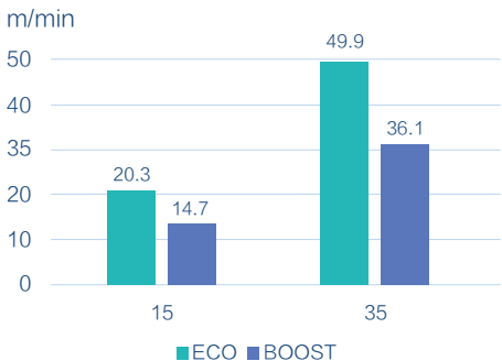
ECO和BOOST的最高运行速度对比
