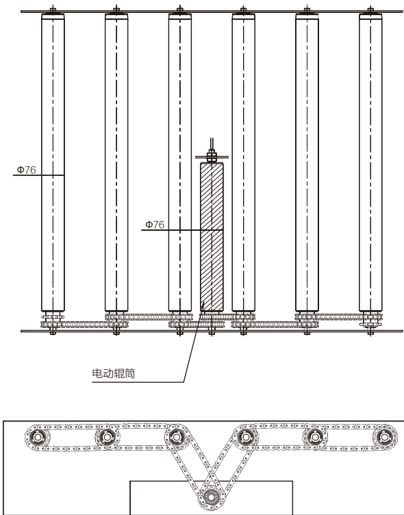
电动辊筒下置式应用示意
